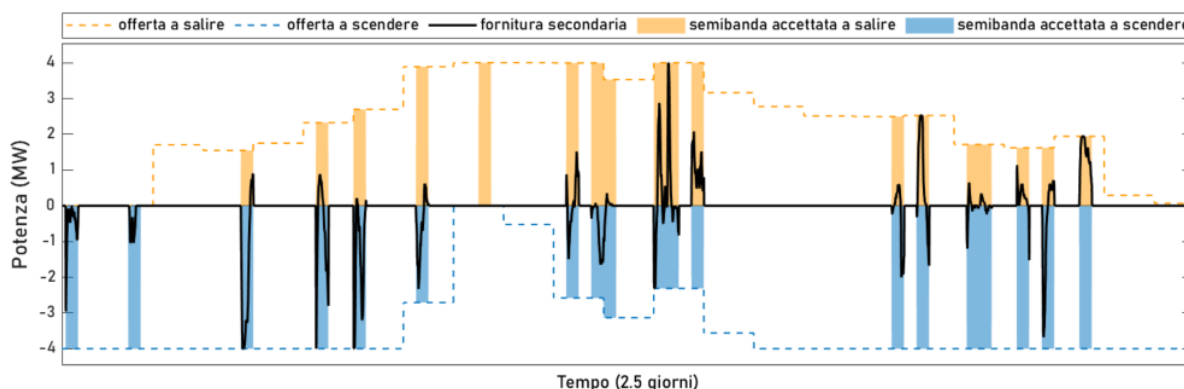
Figura 42 Fornitura di servizio di regolazione secondaria (aFRR)
