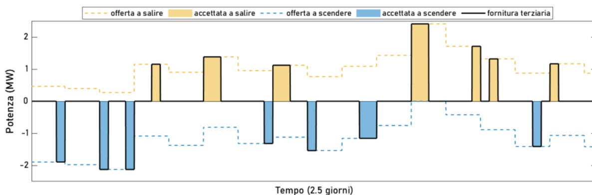
Figura 43 Fornitura di servizio di regolazione terziaria (mFRR)
