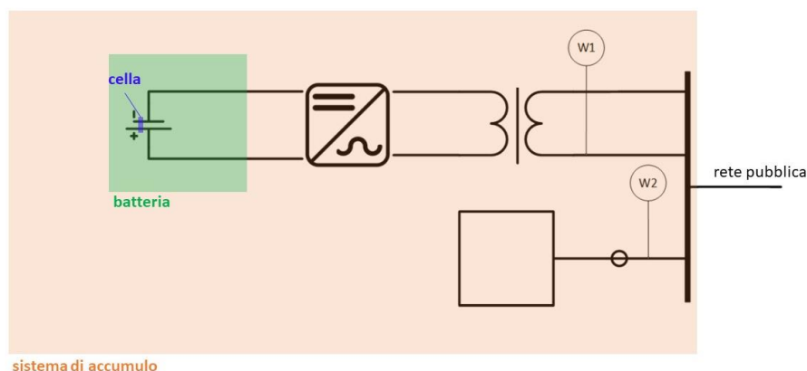
Figura 2 Classificazione modelli matematici batterie rispetto al sistema considerato
